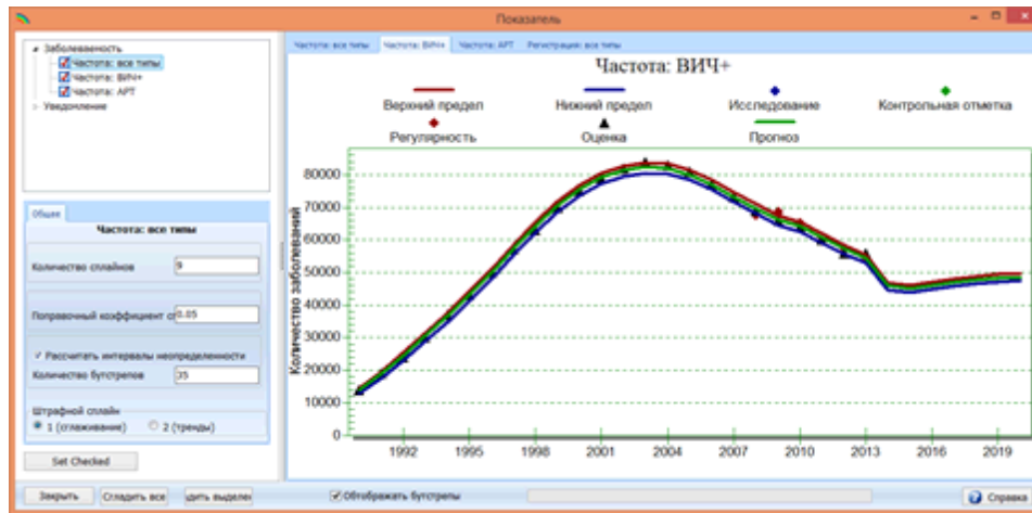
Рисунок 7. Подгонка заболеваемости ТБ среди ВИЧ+ индивидуумов
